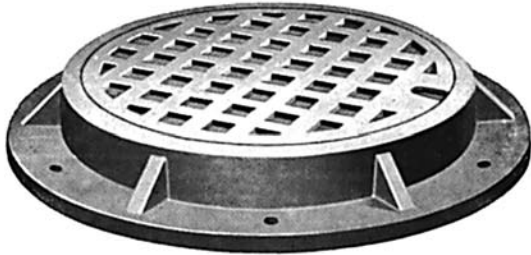
R-1647 Manhole Frame & Solid Lid
